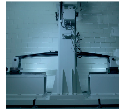
Тестирование рессоры
